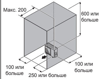
(2) Препятствия сзади, выше и по бокам
