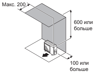
(1) Препятствия сзади и выше
