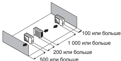
(1) Размещение модулей в одну параллель
