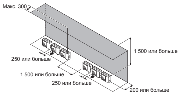
Препятствия сзади и выше
