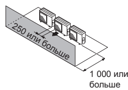
(2) Препятствия только спереди
