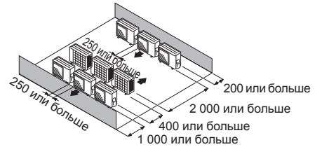
(2) Размещение модулей в несколько параллелей
