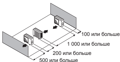
(1) Размещение модулей в одну параллель
