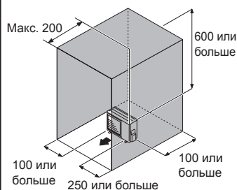
(2) Препятствия сзади, выше и по бокам
