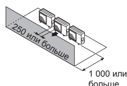
(2) Препятствия только спереди
