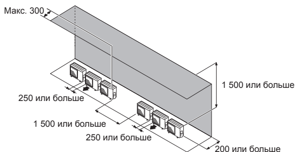
(1) Размещение модулей в одну параллель
