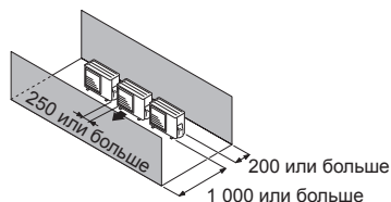
(3) Препятствия спереди и сзади
